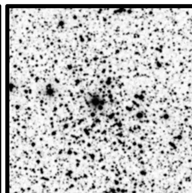
NGC 6834 7'
