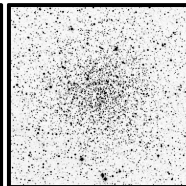
NGC 6791, Berk 46 15'
