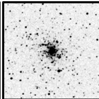
NGC 6342 5'
