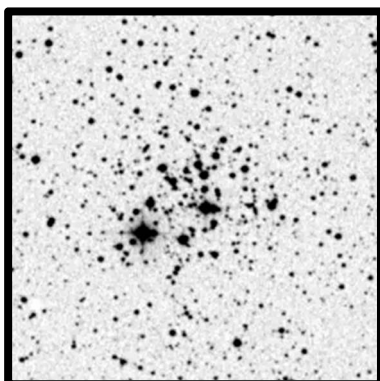
NGC7128 7'
