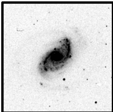
NGC 5248 8'
