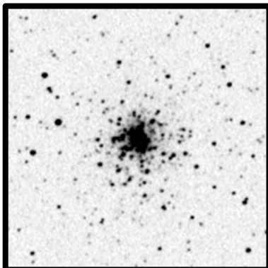
NGC 6284 5'
