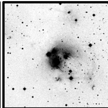
NGC7129 10'
