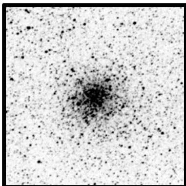
NGC 6553 7'
